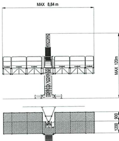
CROQUIS MONOCOLUMNA CAMAC-2000
