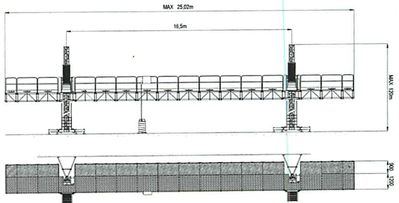
CROQUIS BICOLUMNA CAMAC-2000
